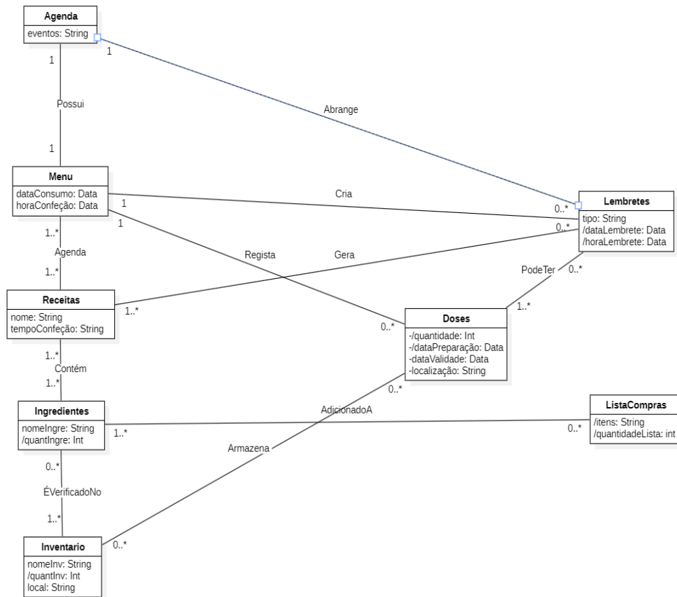
Figura 2- Modelo de Domínio
